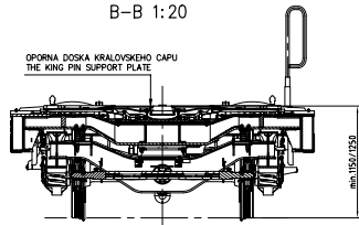
B-B 1:20
